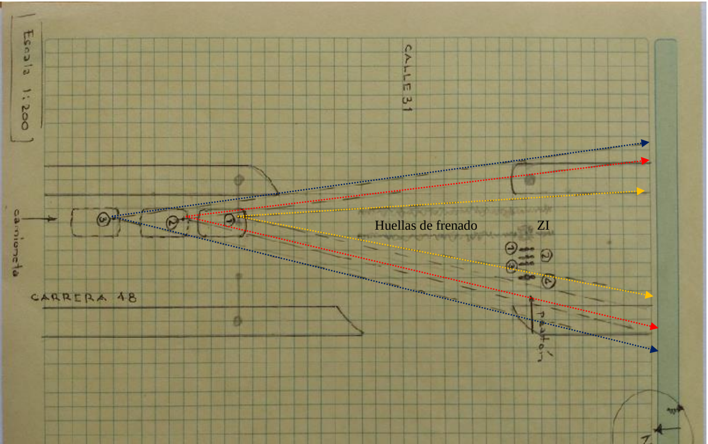
Diagrama Posición-Velocidad en el que se ubican las posiciones del peatón y de la camioneta simultáneamente respecto de la zona de impacto ZI. Entre las flechas punteadas se aprecian los campos visuales del conductor en las posiciones (1), (2) y (3) de su trayectoria.
