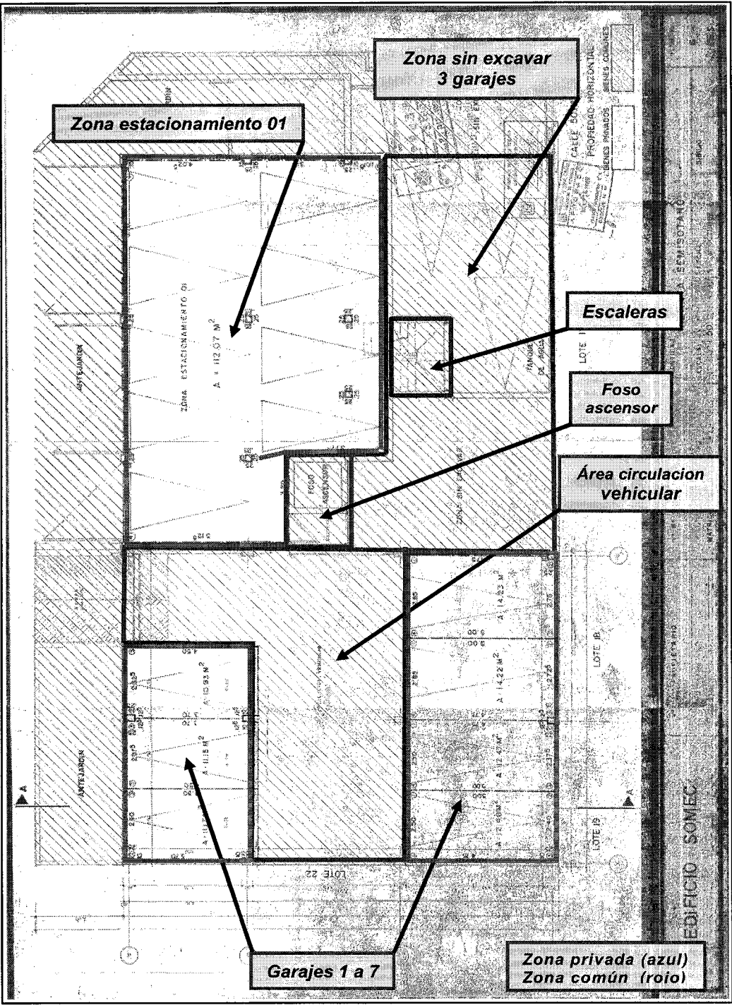
Ilustración 3. Planta semisótano.
