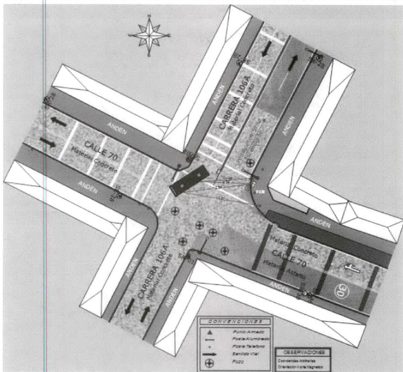
Imagen 11. Plano Topográfico 33494 elaborado a escala, en el cual se detalla únicamente la ubicación de la buseta de placa VEY 824, acotada por el personal investigativo de FCII.
