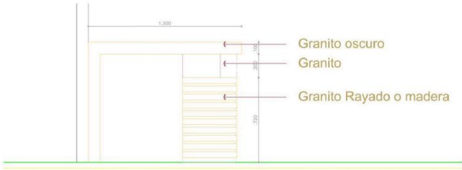
VISTA B-B
