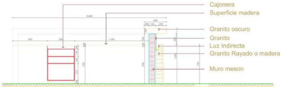
VISTA C-C
