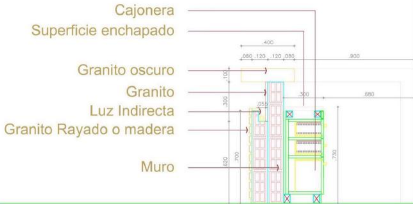
VISTA D-D
