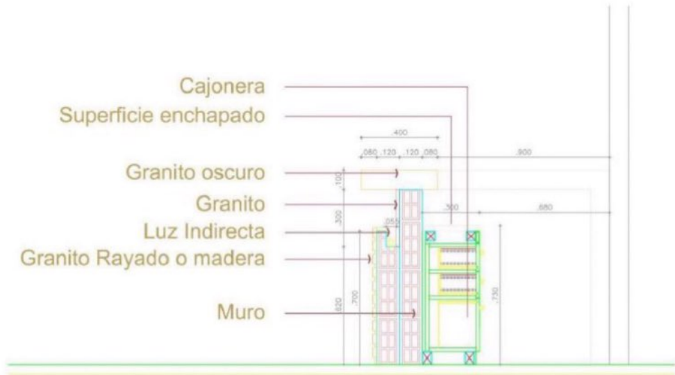
VISTA D-D
