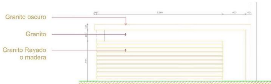
VISTA A-A
