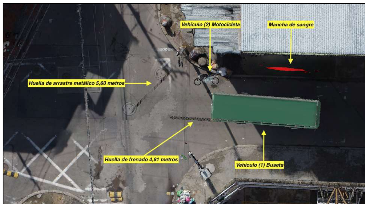
Imagen 26. Localización de los elementos materia de prueba registrados en el plano topográfico una vez realizado el procesamiento de sobrexposición con el ortomosaico.
