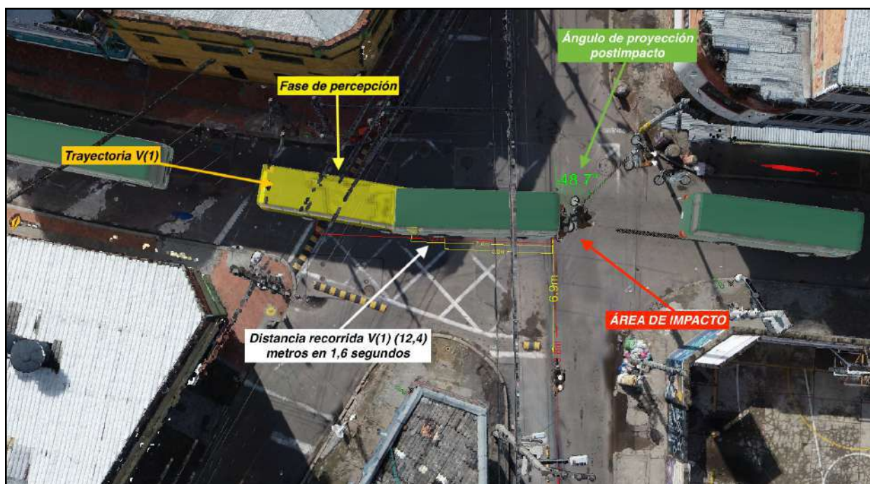
Imagen 42. Reconstrucción en tres dimensiones de la dinámica del accidente en vista cenital, se señalan la trayectoria pre impacto de la buseta, fase de percepción de riesgo del conductor y área de impacto.
