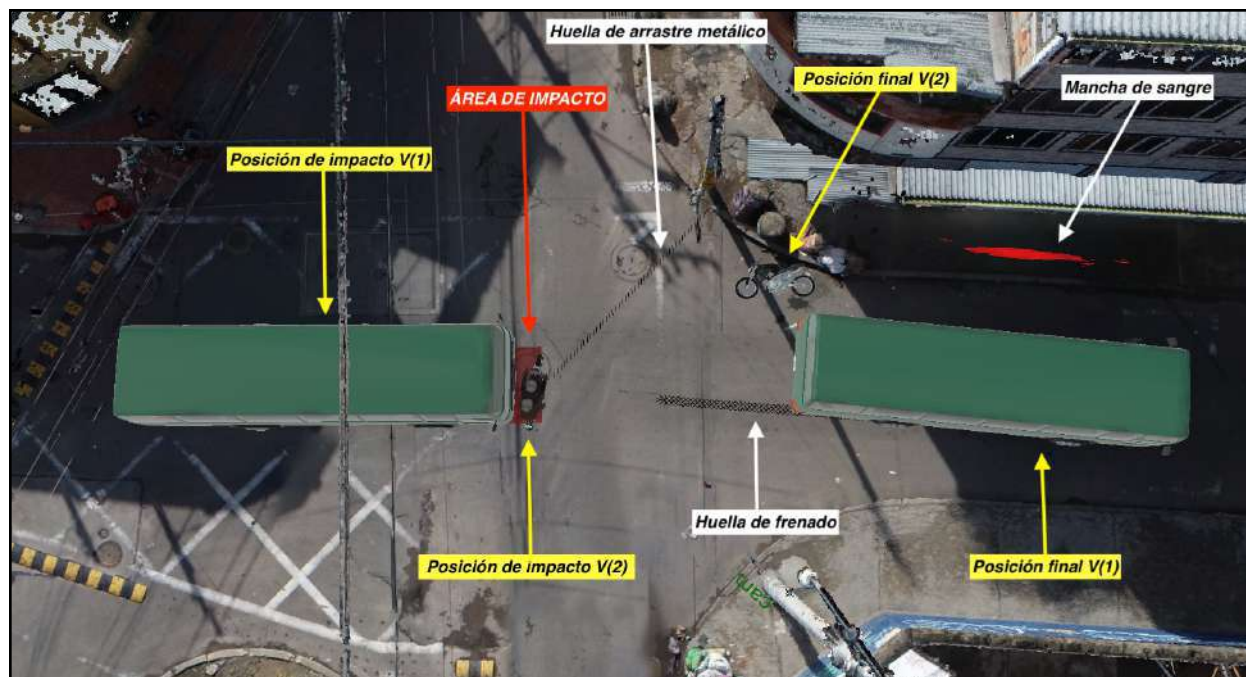
Imagen 41. Reconstrucción en tres dimensiones área de impacto en correlación con las evidencias fijadas en el plano topográfico y posiciones finales.
