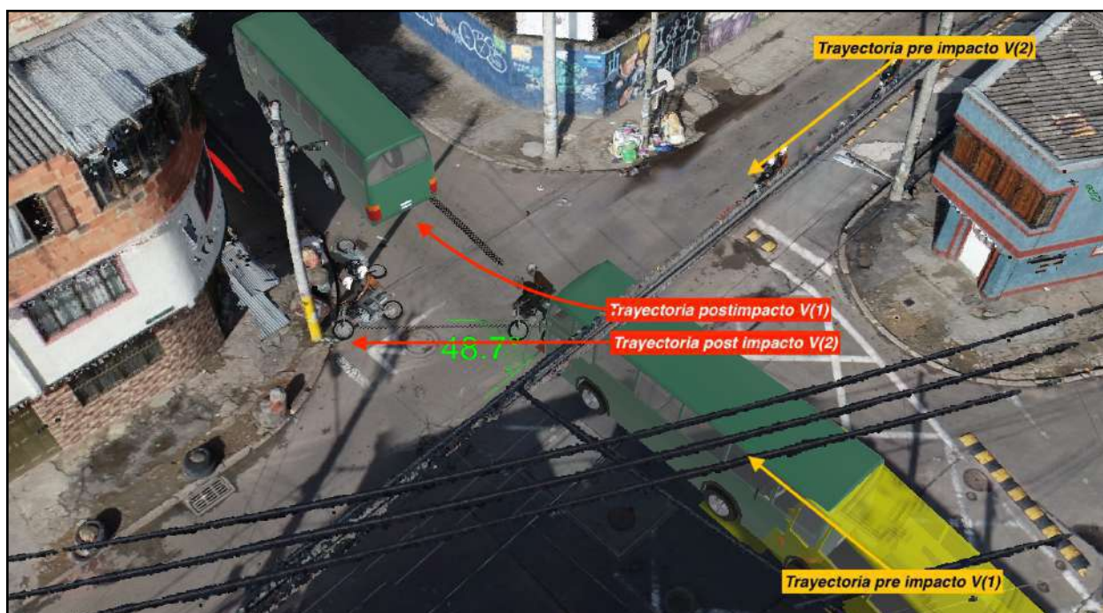
Imagen 43 Reconstrucción en tres dimensiones de la dinámica del accidente se señalan las trayectorias pre impacto, y postimpacto.
