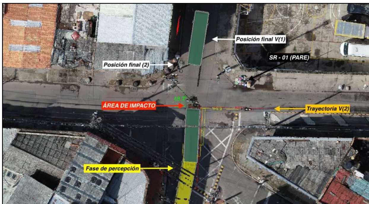
Imagen 43 Reconstrucción en tres dimensiones de la dinámica del accidente vista cenital, se señala la trayectoria pre impacto del V(2), señal de PARE en la diagonal 51A sur, posiciones finales de los vehículos posterior al impacto y área de impacto.
