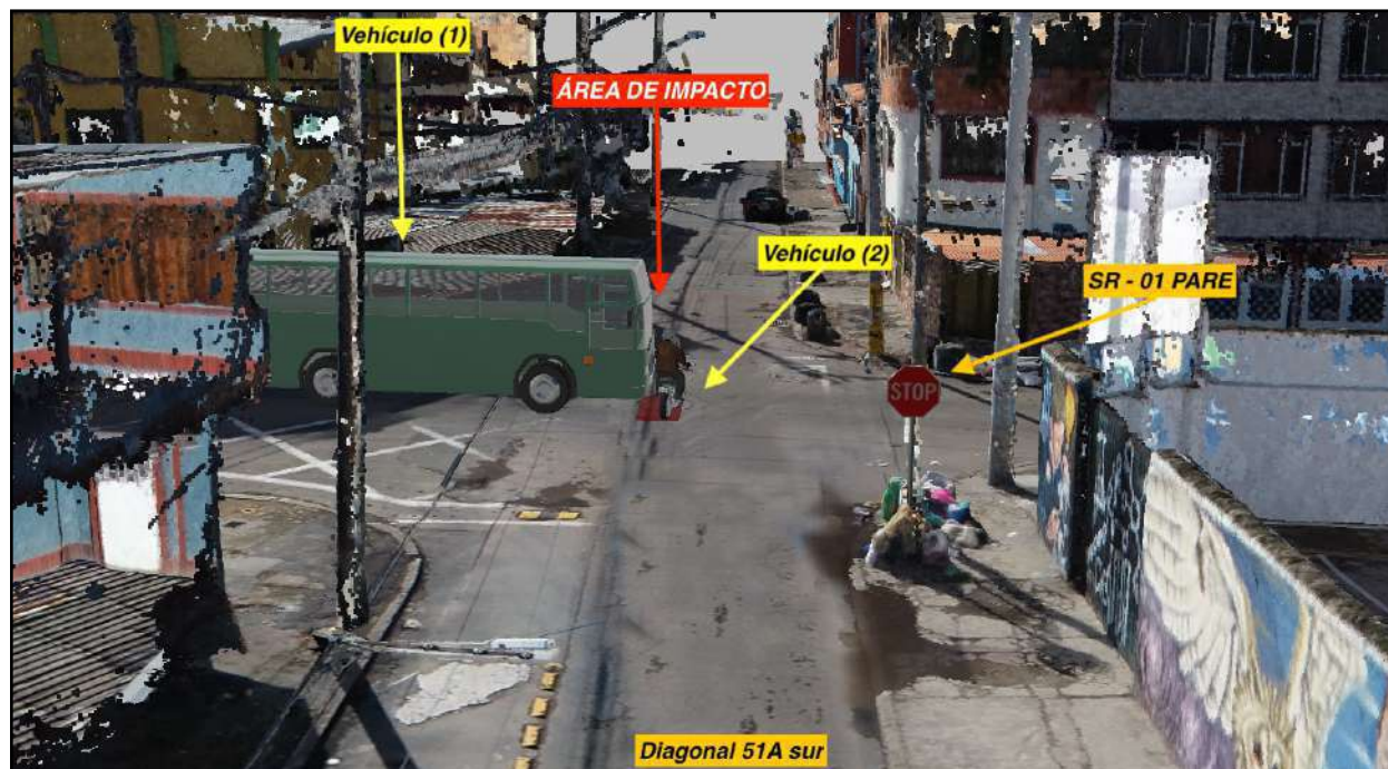
Imagen 40. Reconstrucción en tres dimensiones del área de impacto, vista desde la Diagonal 51A sur, vía por donde viajaba el vehículo (2) motocicleta, se señala la presencia de señal SR - 01 PARE.
