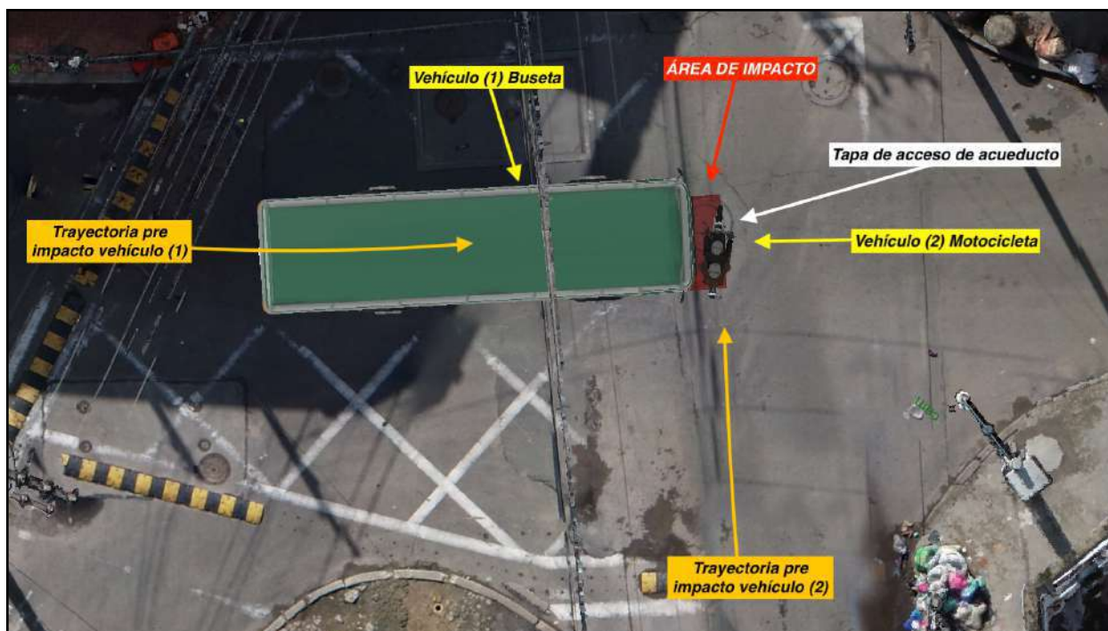
Imagen 38. Reconstrucción en tres dimensiones del área de impacto localizada sobre la tapa de acceso de acueducto en el carril en la Diagonal 51A sur sentido norte a sur.
