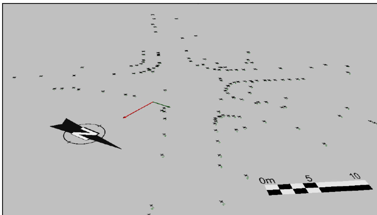
Imagen 3. Nube de puntos de Información topográfica de la vía, obtenida por medio de estación total Nikon Nivo 5.C, procesada con software FaroZone3D.
