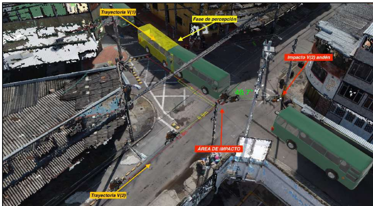
Imagen 43 Reconstrucción en tres dimensiones de la dinámica del accidente se señalan las trayectorias pre impacto, área de impacto, fase de percepción, e impacto de la motocicleta contra el andén en proyección de ángulo de 48,7° postimpacto.
