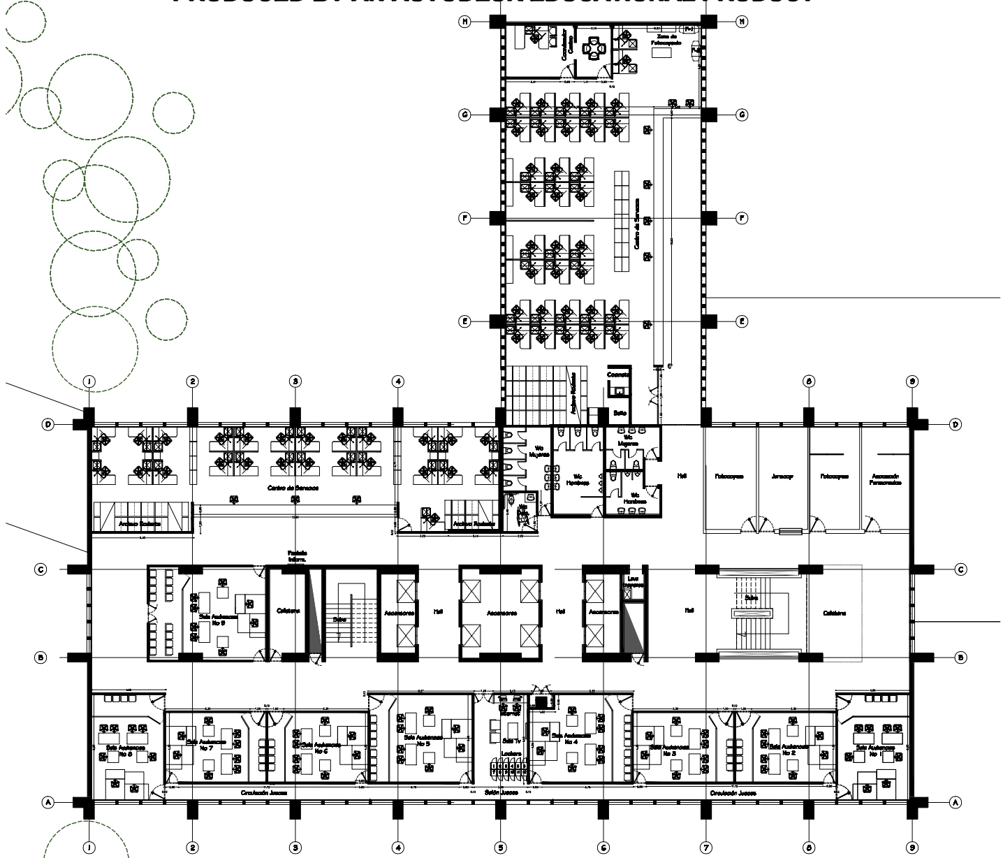
DISEÑO ARQUITECTÓNICO - EDIFICIO JOSE FELIX RESTREPO PISO - 2
