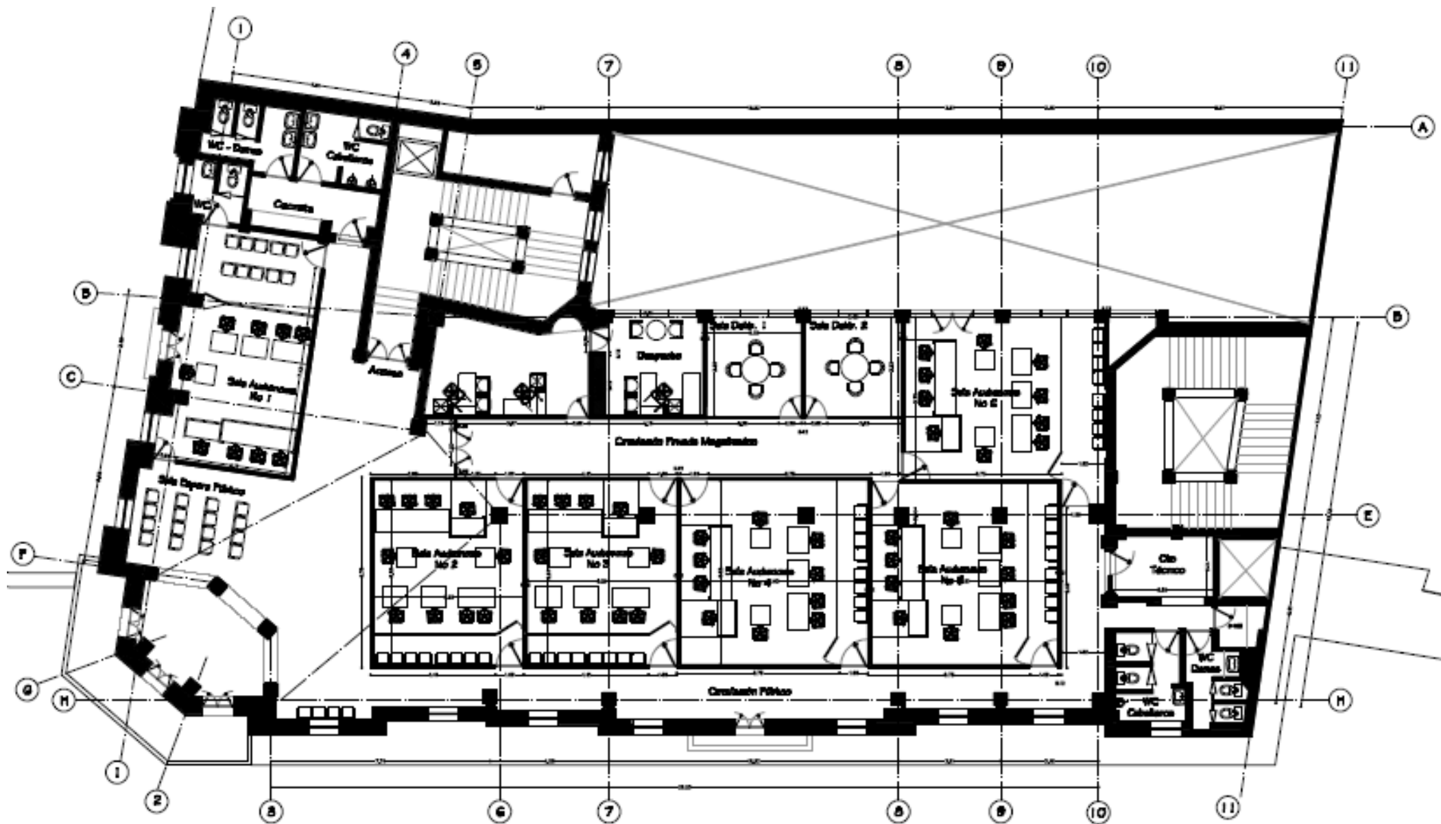
DISEÑO ARQUITECTÓNICO - EDIFICIO OTERO PISO - 2
