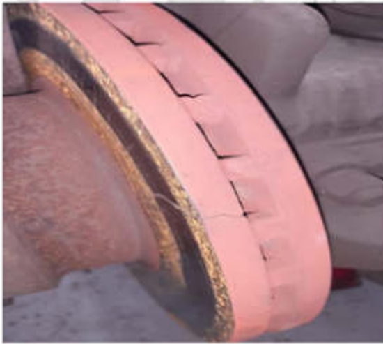
DISCOS DE FRENO FRACTURADOS
