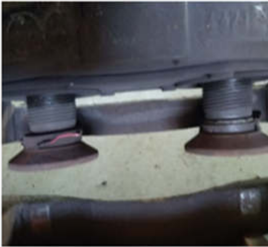
DESPLAZAMIENTO NO UNIFORME EN PISTONES DE MORDAZA
