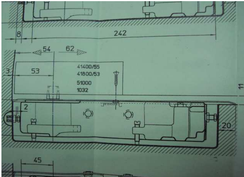
Imagen No. 5 – Imagen de la bisagra hidráulica M60/HD SPEEDY Dimensiones con referencia al pivote
