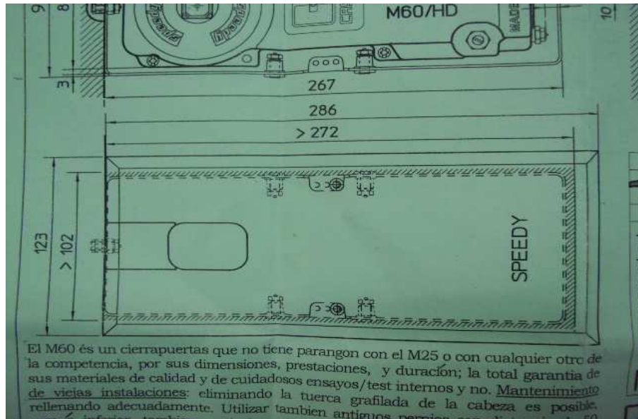
Imagen No. 6 – Tapa de la bisagra hidráulica M60/HD SPEEDY Dimensiones con referencia al pivote
