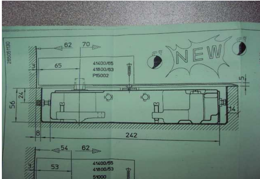
Imagen No. 4 – Longitudes de la bisagra hidráulica M60/HD SPEEDY
