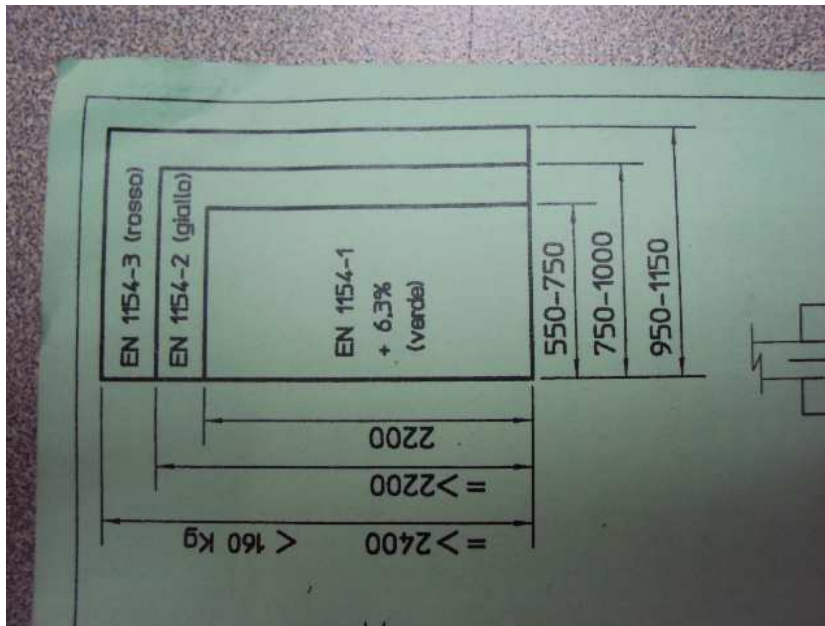
Imagen No. 7– Otras especificaciones de la bisagra hidráulica M60/HD SPEEDY
