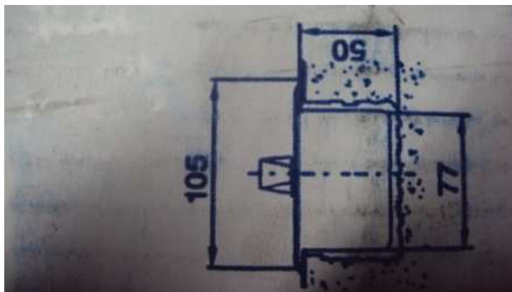
Imagen No. 2 – Ancho y alto de la bisagra hidráulica sevax modelo minus
