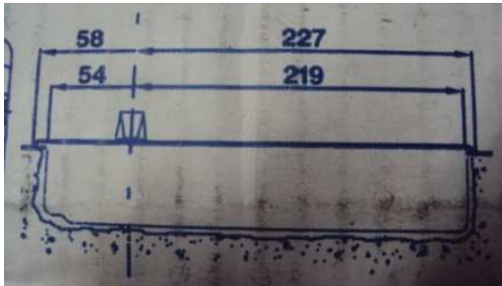
Imagen No. 1 – Longitudes de la bisagra hidráulica sevax modelo minus
