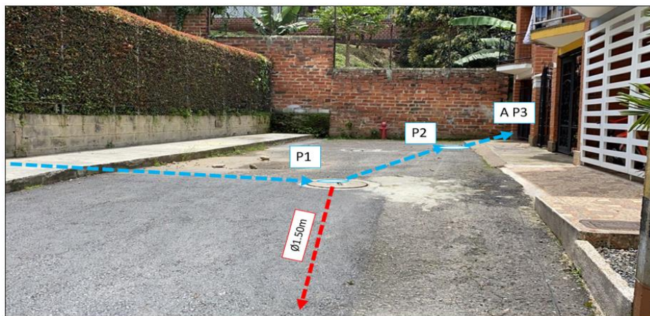
Imagen 10. Punto conexión Aliviadero Ø 1.50 m en P1. Cra 59BB.
