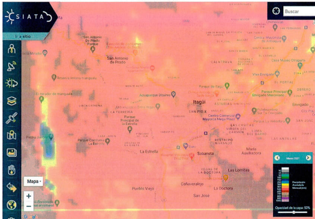
Imagen 4. Mapa Radar del Mes de marzo 2021.
